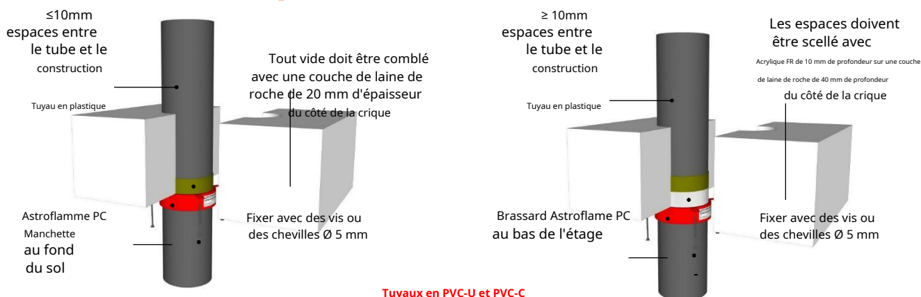
Tuyaux en PVC-U et PVC-C
